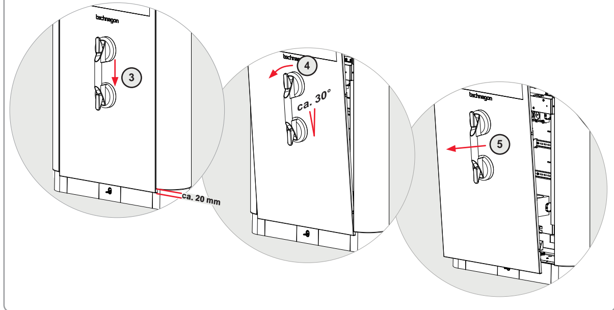
Abbildung 11: Gehäuse öffnen Technagon TEP8 – Anlagen mit abnehmbarer Frontblende
