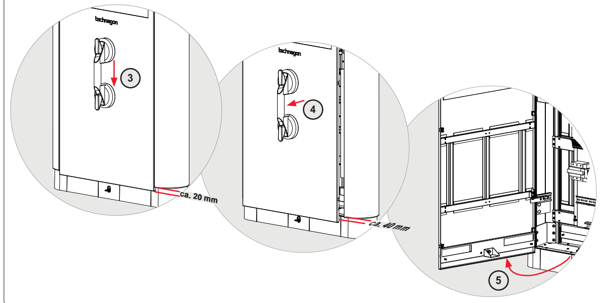
Abbildung 12: Gehäuse öffnen Technagon TEP8 – Anlagen mit schwenkbare Tür
