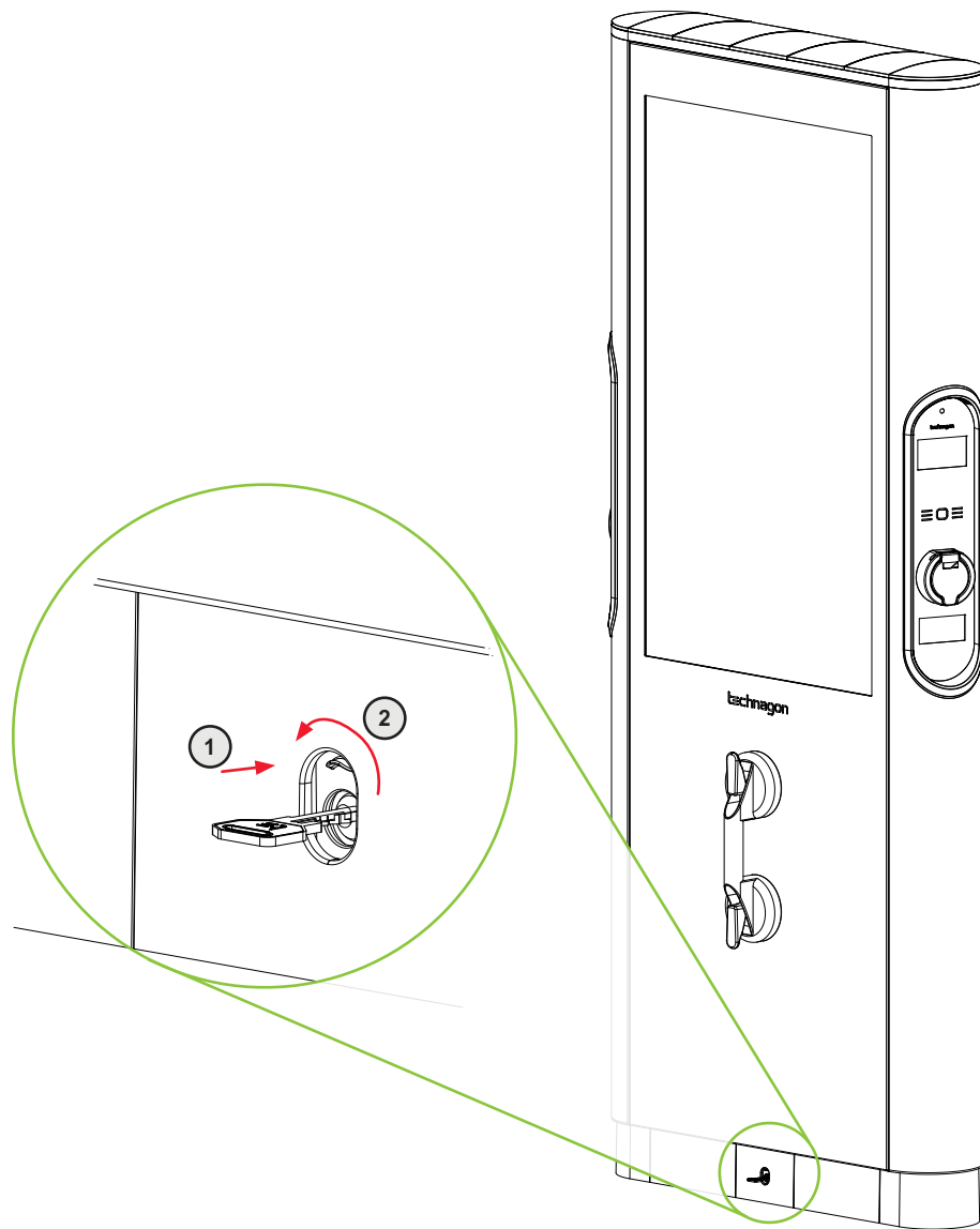
Abbildung 10: Gehäuse öffnen Technagon TEP8 – Frontblende/Türe entriegeln
