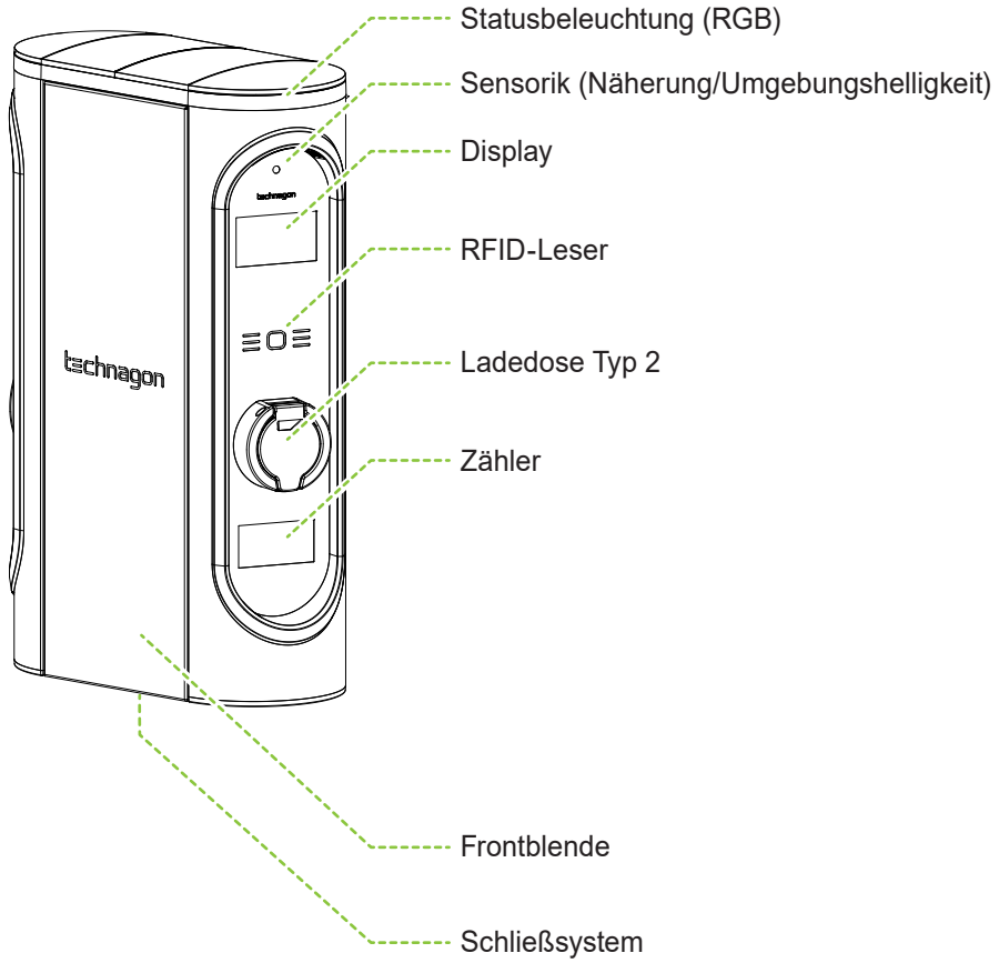
Abbildung 1: Aufbau TEW4 außen
