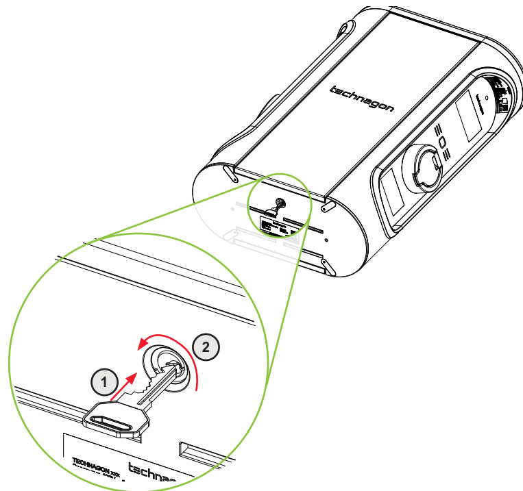
Abbildung 9: Gehäuse öffnen – Frontblende entriegeln
