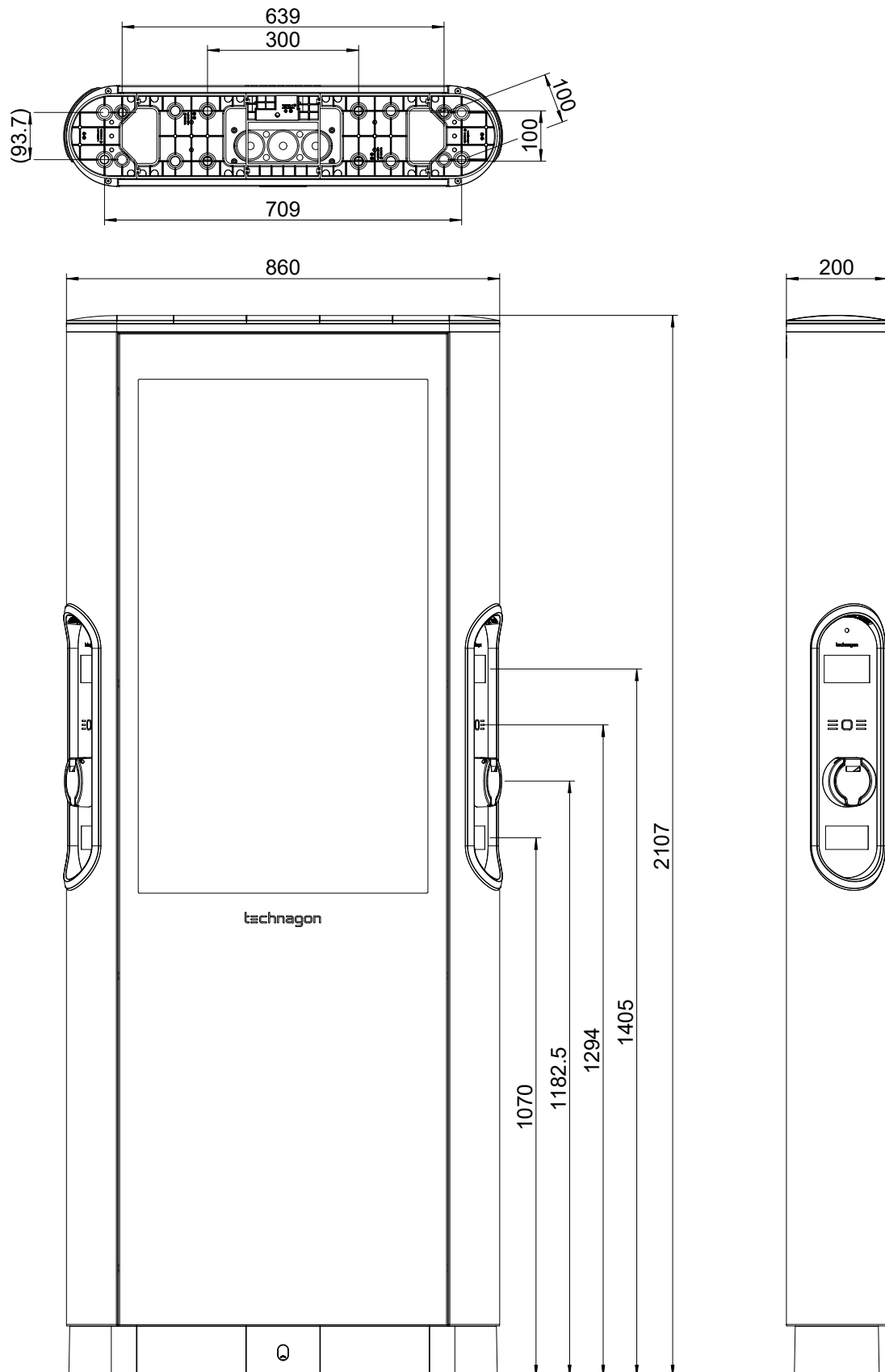
Abbildung 11: Maße Technagon TEP8
