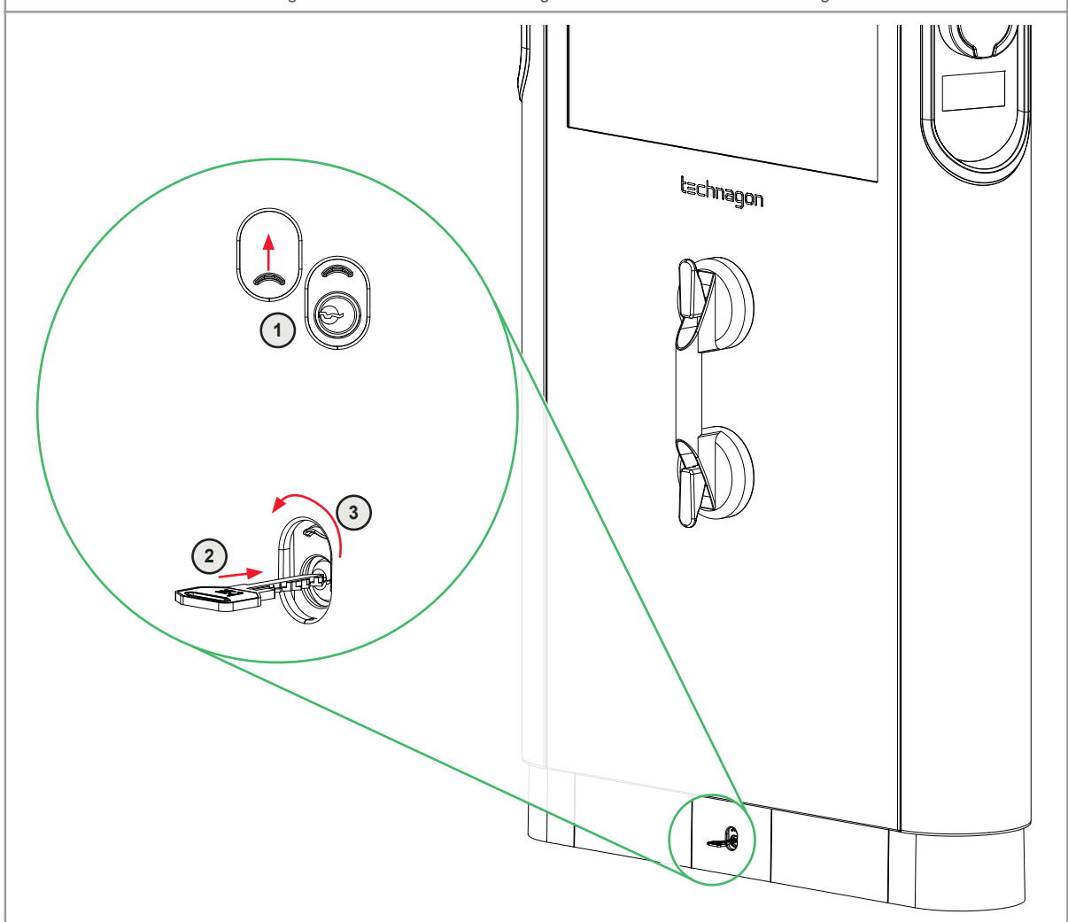
Abbildung 13: Gehäuse öffnen Technagon TEP8 – Frontblende/Türe entriegeln
