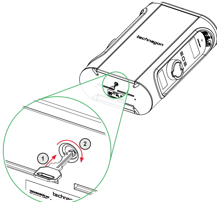
Abbildung 12: TEW4 Gehäuse öffnen – Frontblende entriegeln
