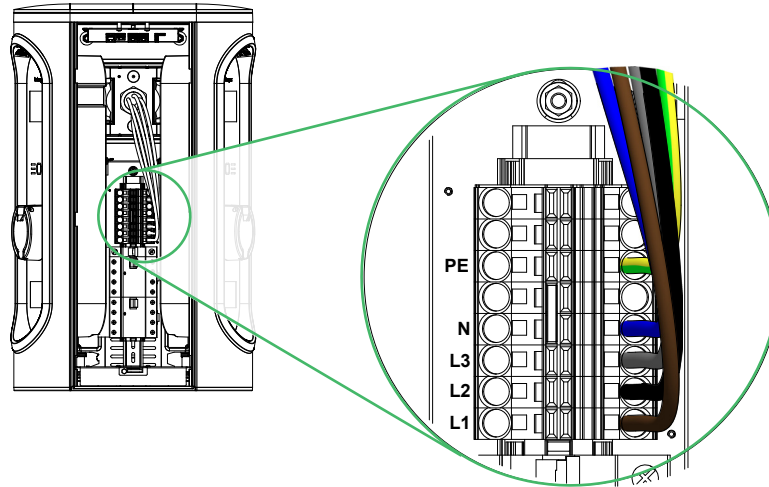
Abbildung 17: Zuleitung anschließen
