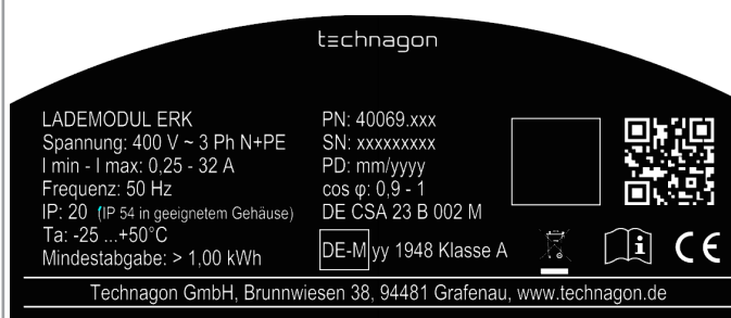
Abbildung 2: Typenschild Technagon Lademodul
