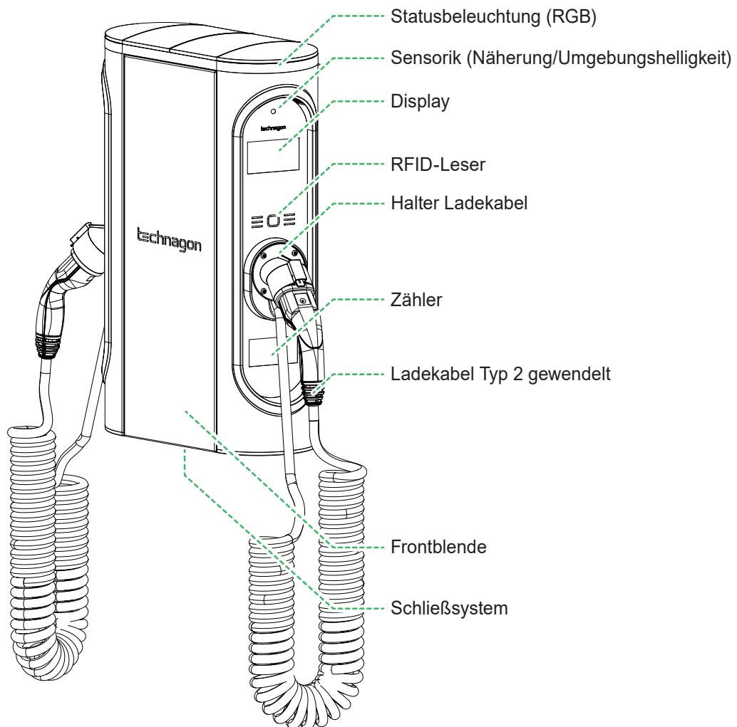
Abbildung 5: Aufbau TEW4 mit Kabel
