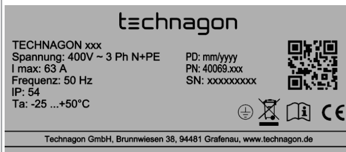
Abbildung 1: Typenschild Technagon TEW4
